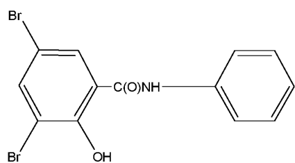
dibromosalalan
