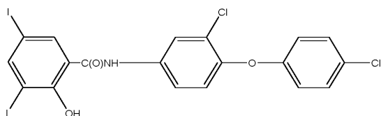
rafoxanide
