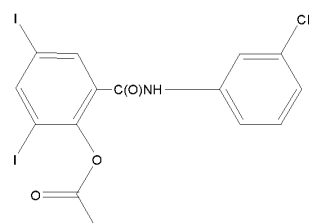
clioxanide
