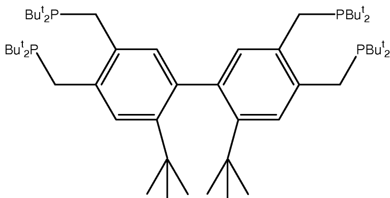
1,2-bis(di-tert-butyl(phosphinomethyl))-4-tertbutyl-5-(2'-tertbutyl-4',5'-bis(di-tert-butyl(phosphinomethyl))phenyl)benzene
