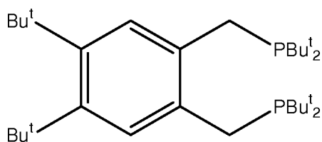
1,2-bis(di-tert-butyl(phosphinomethyl))-4,5-di-tert-butylbenzene
