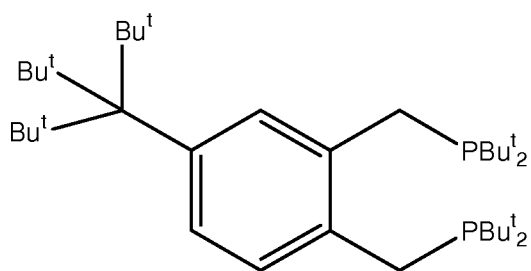
1,2-bis(di-tert-butyl(phosphinomethyl))-4-(tri-tert-butylmethyl)benzene
