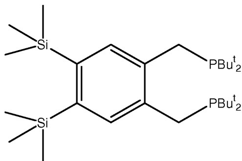
1,2-bis(di-tert-butyl(phosphinomethyl))-4,5-bis(trimethylsilyl)benzene
