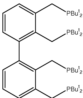
1,2-bis(di-tert-butyl(phosphinomethyl))-3-(2',3'-bis(di-tert-butyl(phosphinomethyl))phenyl)benzene
