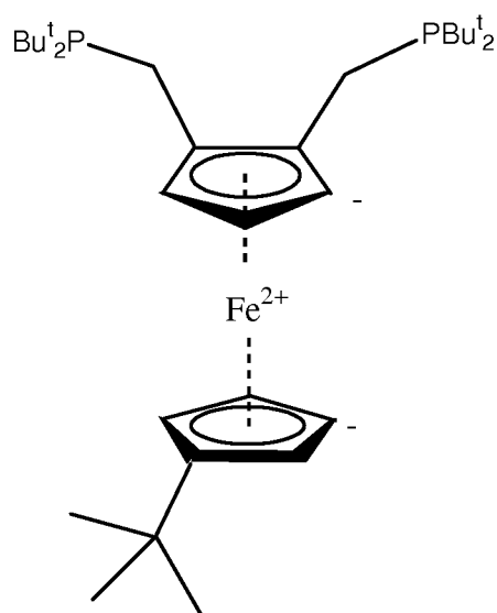
1,2-bis(di-tert-butylphosphinomethyl)-1'-tert-butyl ferrocene
