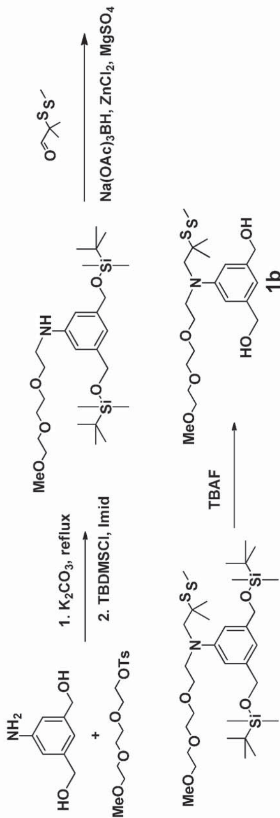
Figure 46. Alternate Synthesis of (5-((2-(2-methoxyethoxy)ethoxy)ethoxy)ethyl)(2-methyl-2-(methyl(disulfanyl)propyl)amino)-1,3-phenylene)dimethanol ( 1b )
