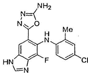
[6-(5-Amino-[1,3,4]oxadiazol-2-yl)-4-fluoro-1H-benzoimidazol-5-yl]-(4-chloro-2-methyl-phenyl)-amine (24b)
