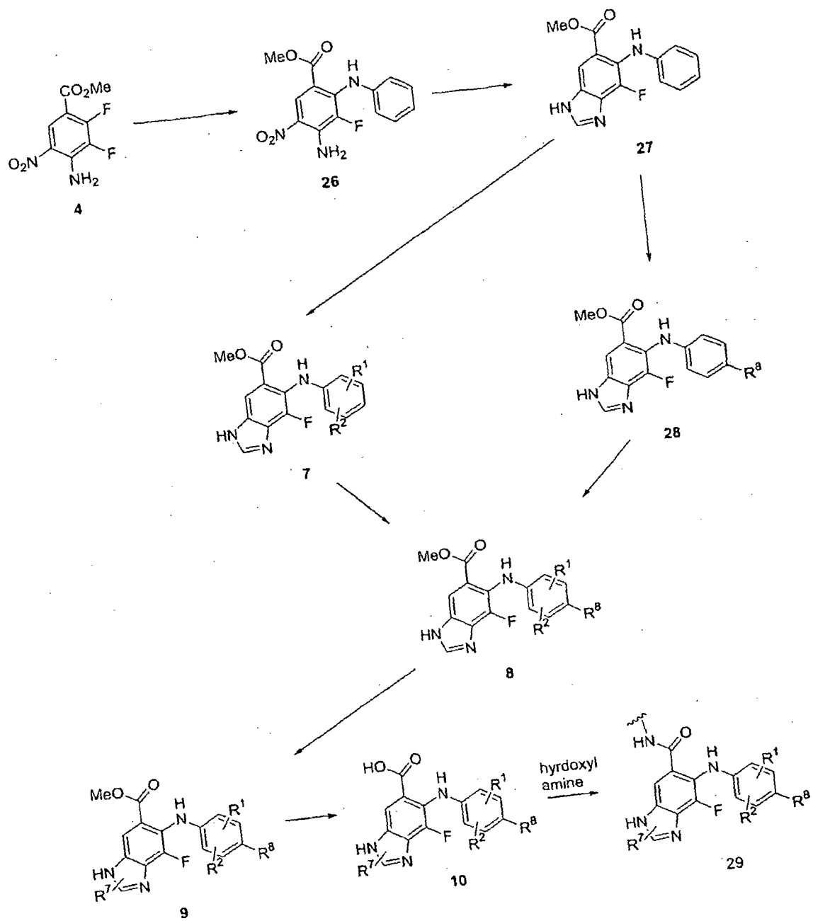
Scheme 1a
