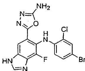
[6-(5-Amino-[1,3,4]oxadiazol-2-yl)-4-fluoro-1H-benzoimidazol-5-yl]-(4-bromo-2-chloro-phenyl)-amine (24c)
