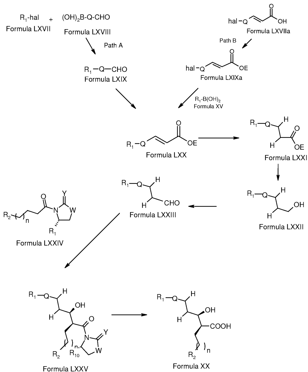
Scheme-VII
