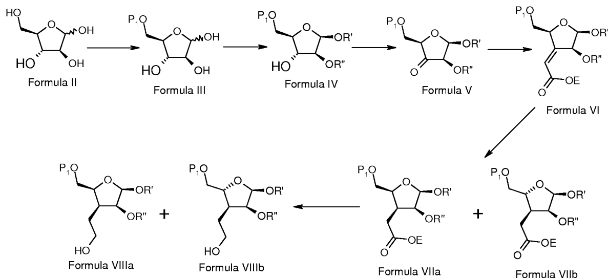
Scheme-I
