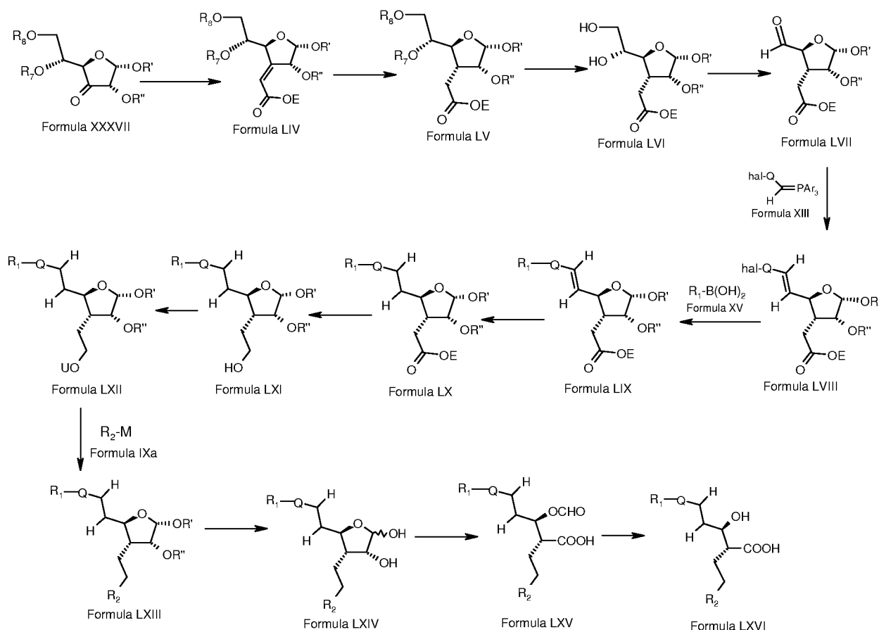
Scheme-VI
