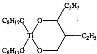
Di(2-ethyl-1-hexyl) 2-ethylhexane-1,3-dioxytitanate
