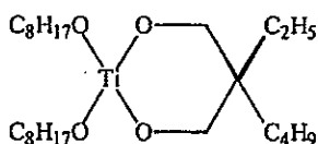
Di(2-ethyl-1-hexyl) 2-(1-butyl)-2-ethylpropane-1,3-dioxytitanate
