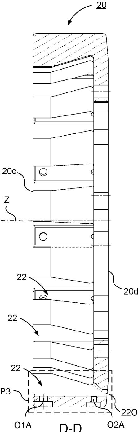
D-D Fig. 9
