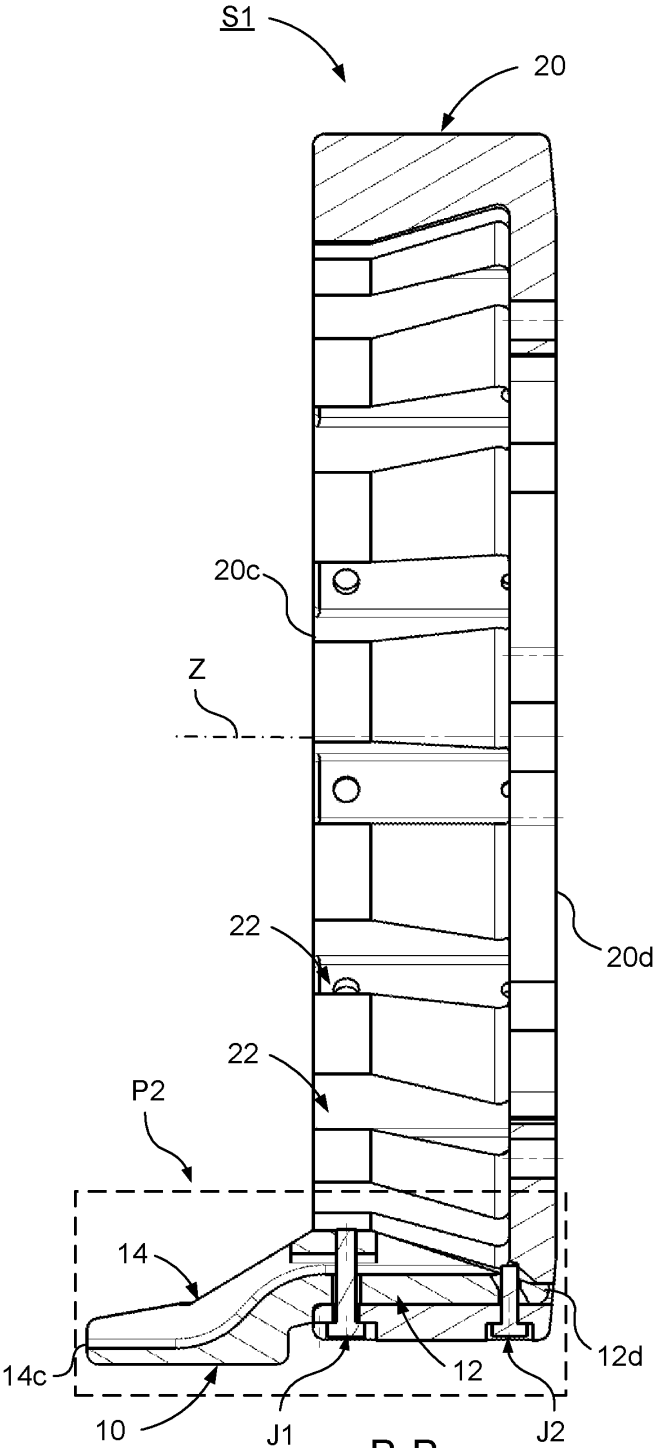
B-B Fig. 8
