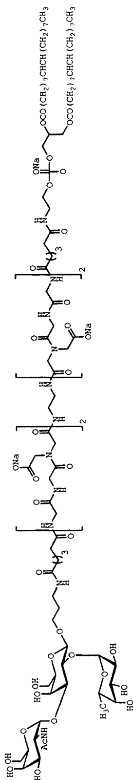
A trr1 -S 1 -S 5 -S 4 -S 5 -DOPE (VI)
