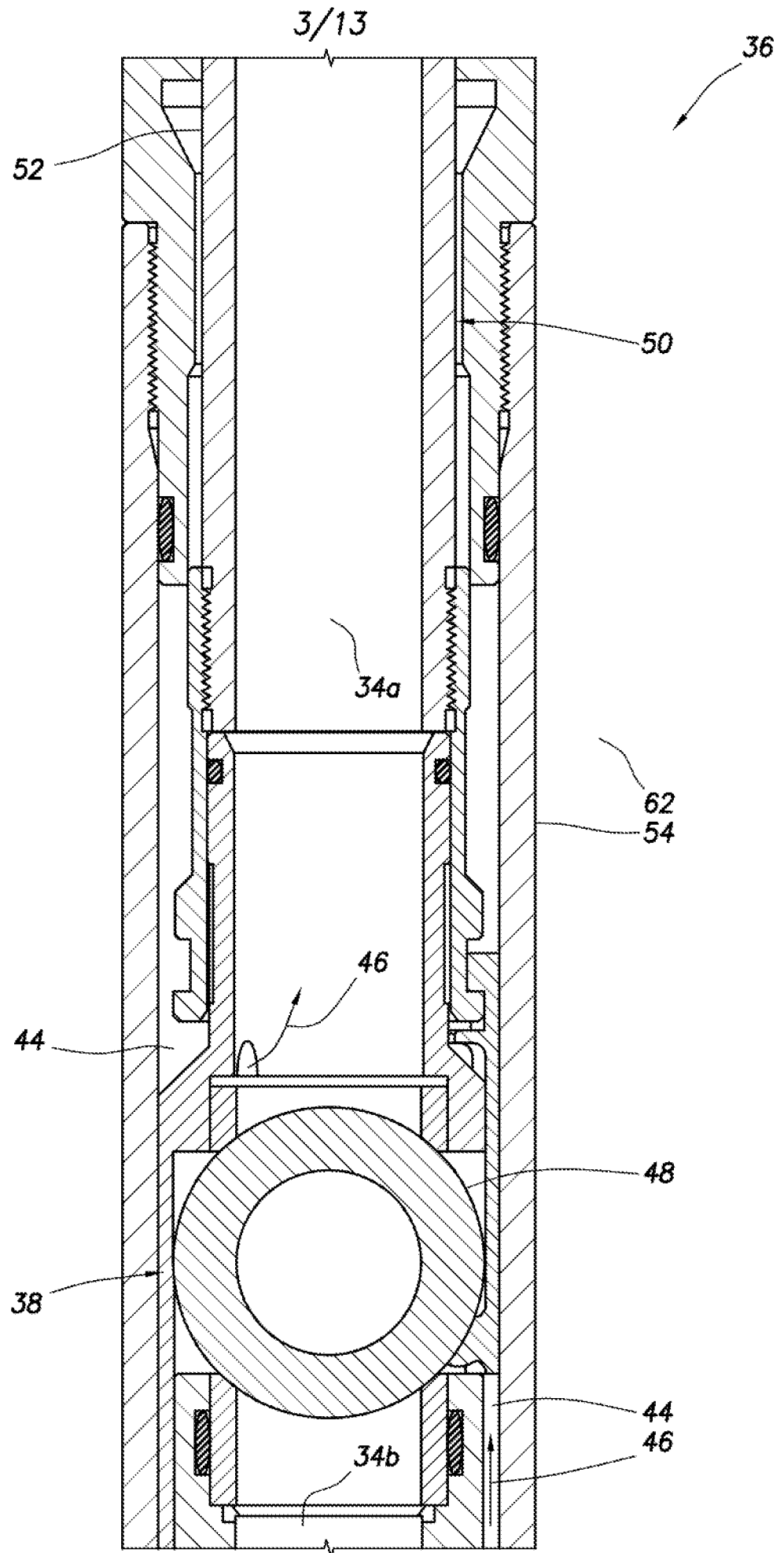
FIG. 2B
