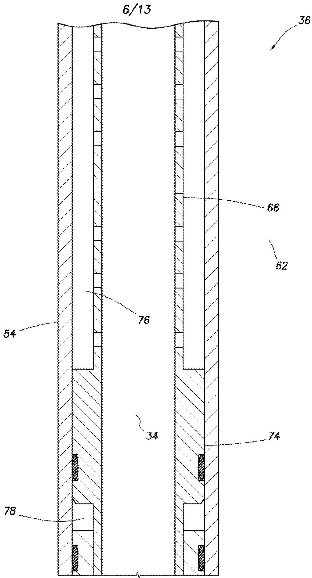
FIG. 2E
