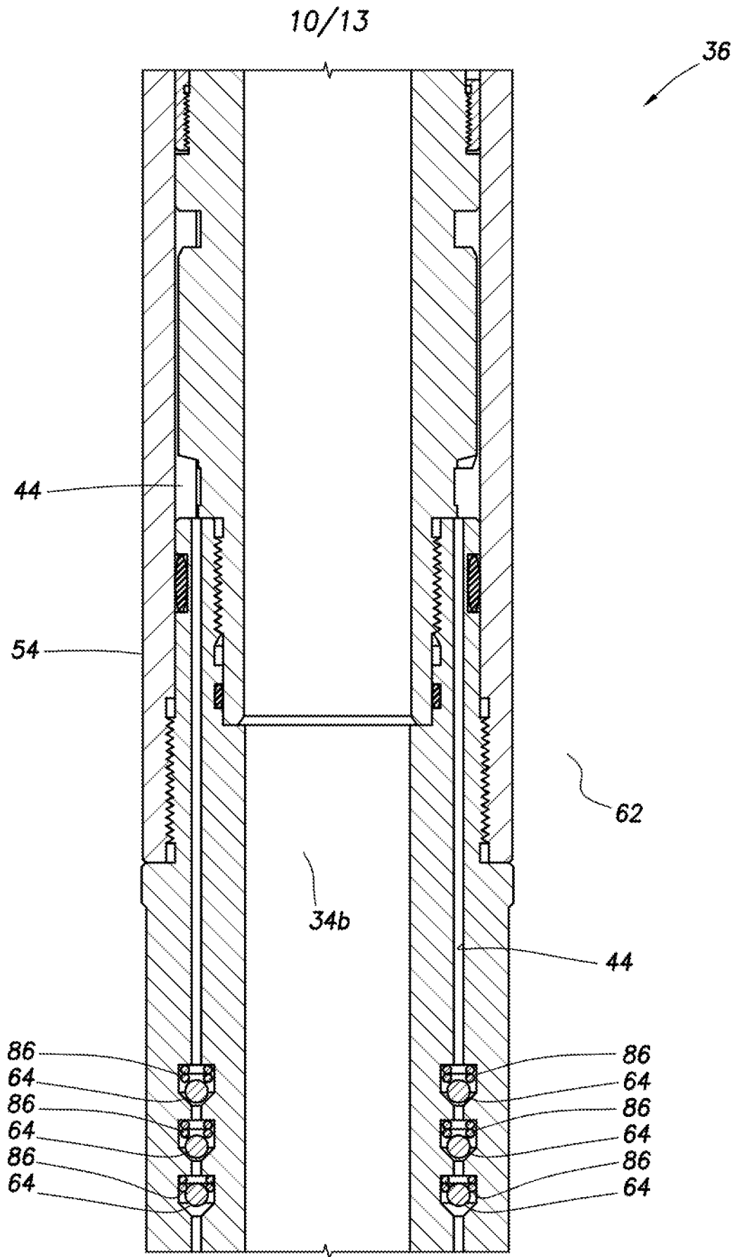
FIG. 3C
