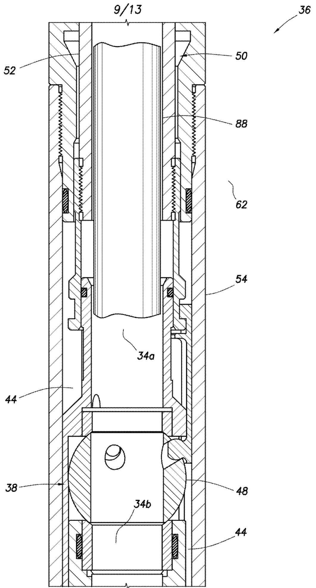
FIG. 3B
