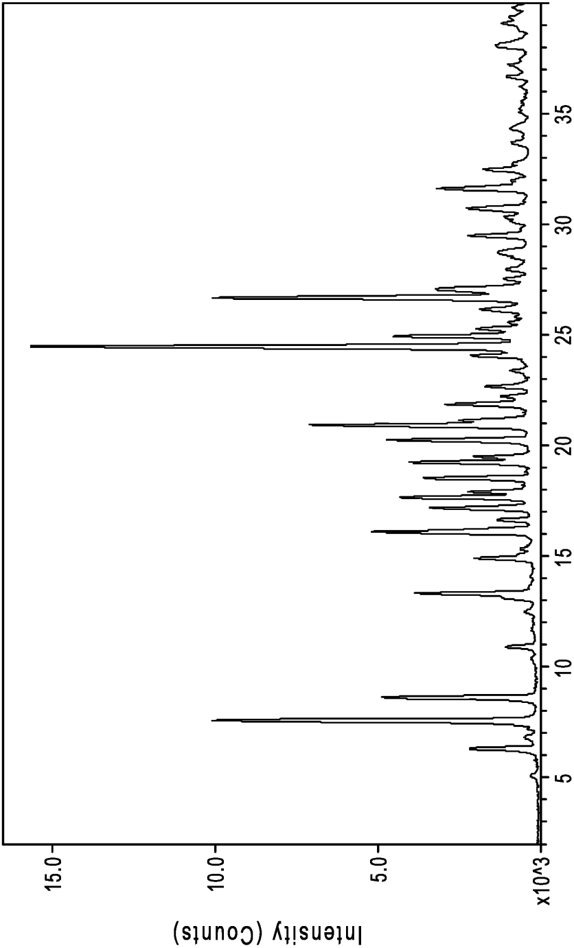
2θ (deg)
