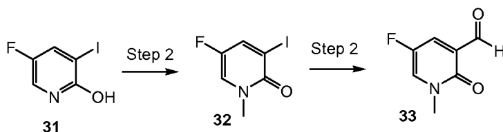
Scheme 10a
