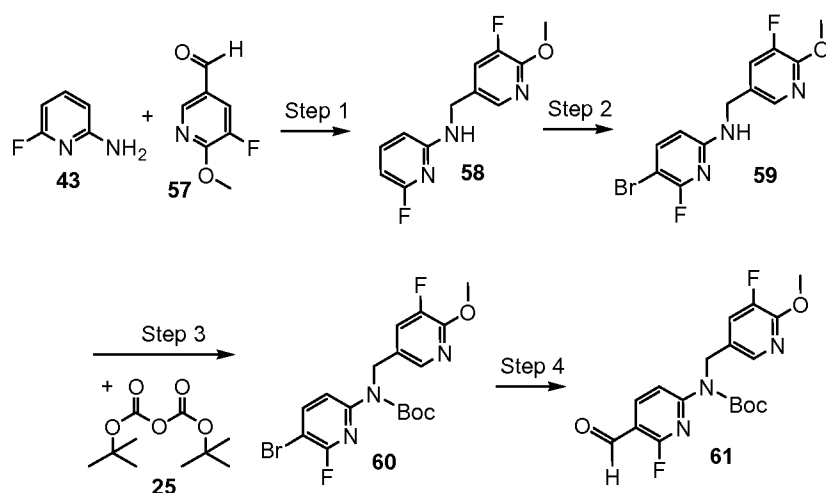
Scheme 10e
