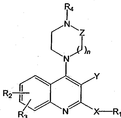
(Ib)
