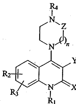
(Ia)
