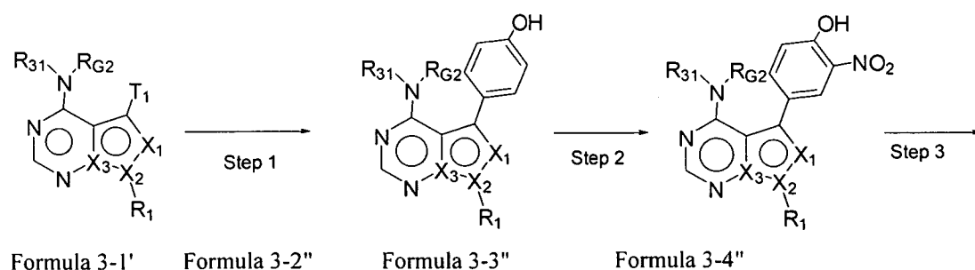
Scheme D'
