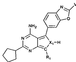
Subclass 12b
