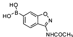
J-4-B
