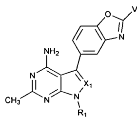
Subclass 2a
