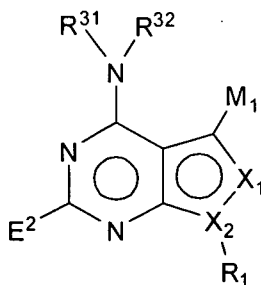
Formula I-A
