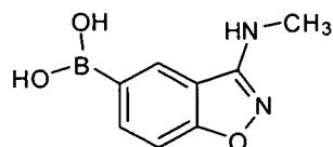
L-6-B
