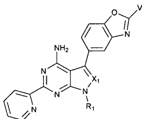
Subclass 8a
