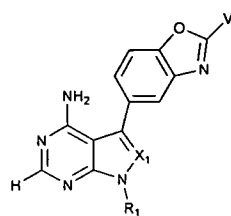
Subclass 1a
