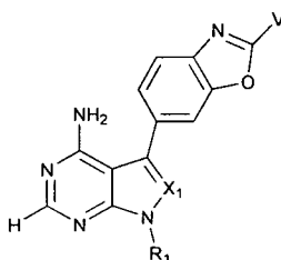
Subclass 9a
