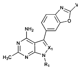
Subclass 10a
