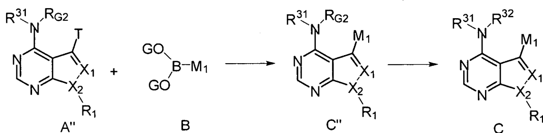
Scheme D'
