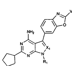
Subclass 12a
