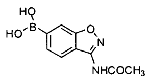
J-4-B
