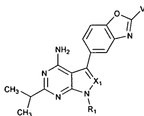
Subclass 3a
