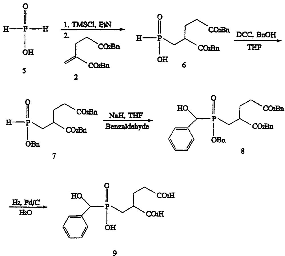
SCHEME VI
