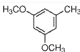
3,5-dimethoxytoluene
