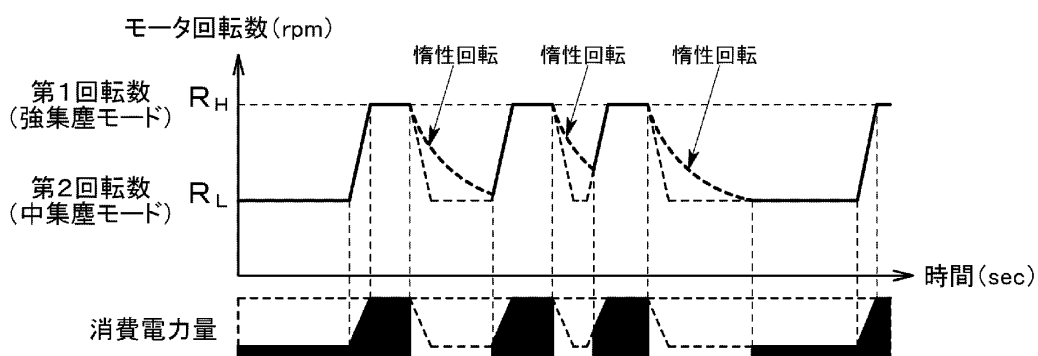
(c) インバータによる回転制御+慣性回転
