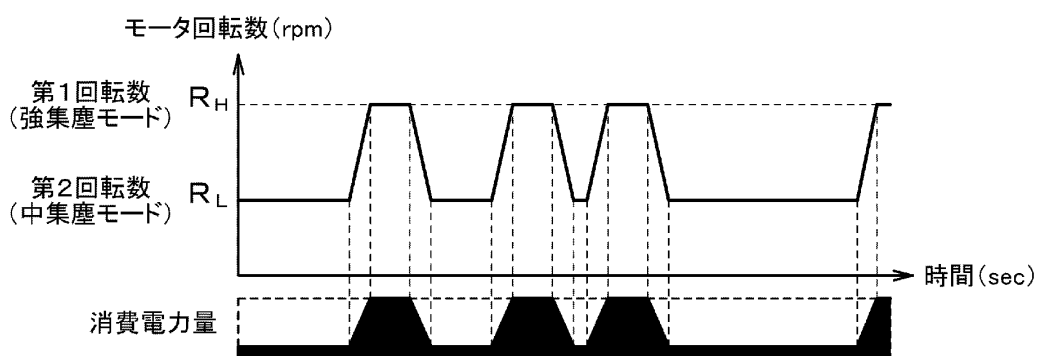
(b) インバータによる回転制御のみ
