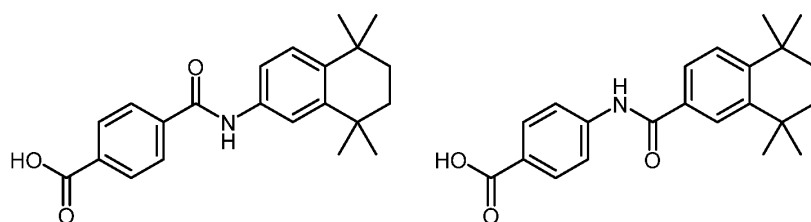
Tamibarotene (AM80)
