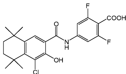
(III) (IRX5183).
