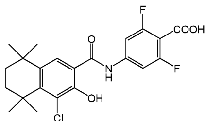
(III) (IRX5183).
