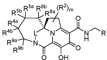
Formula VIa;
