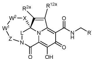
Formula Va.
