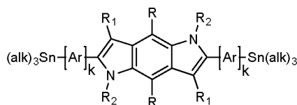
1a precursor
