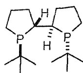
(SSRR)-TangPhos
