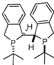
(+)-DuanPhos
