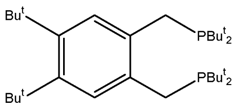
1,2-bis(di-tert-butyl(phosphinomethyl))-4,5-di-tert-butyl benzene
