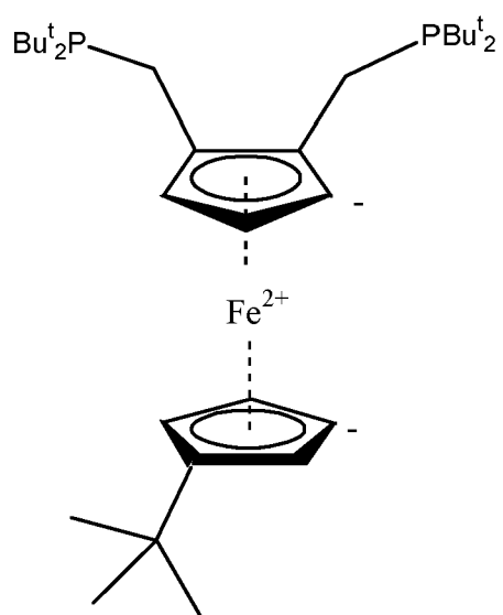
1,2-bis(di-tert-butylphosphinomethyl)-1'-tert-butyl ferrocene
