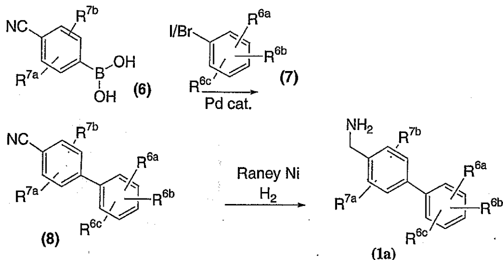
SCHEME 2a
