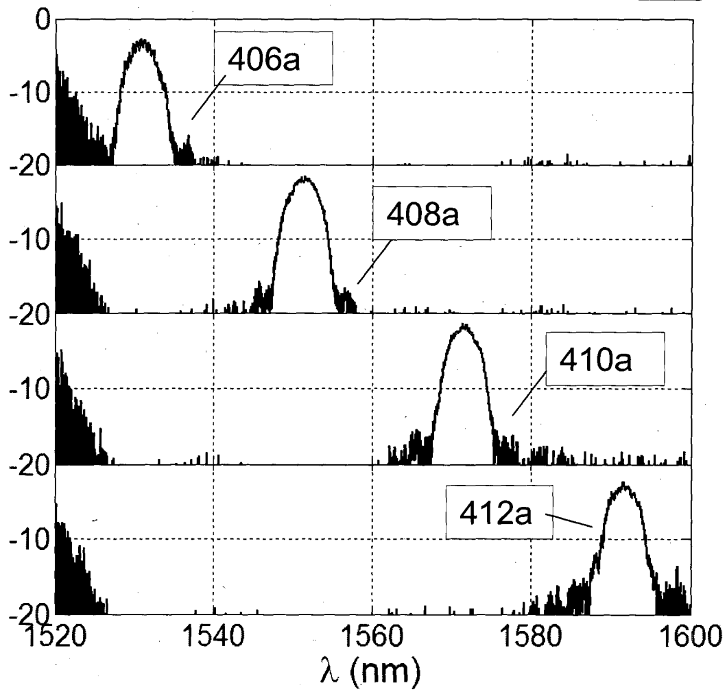
FIG. 4I
