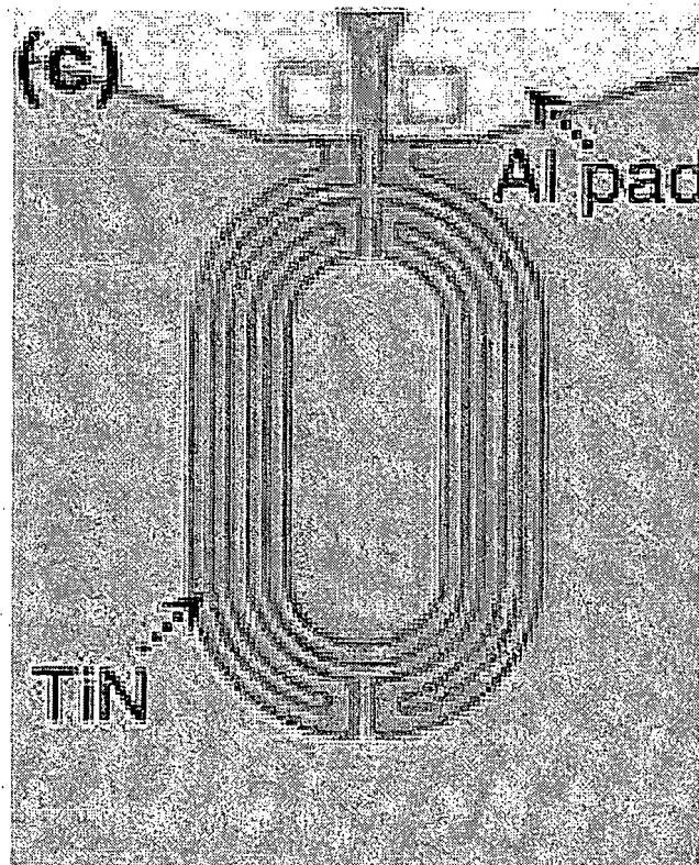
FIG. 5C
