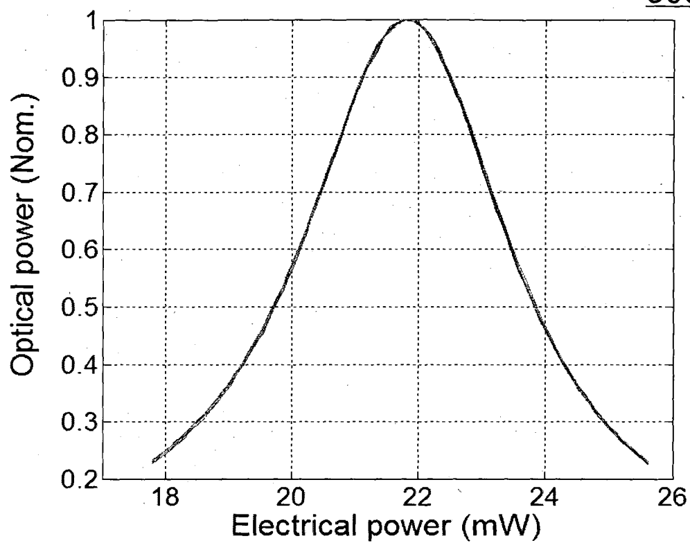
FIG. 5G
