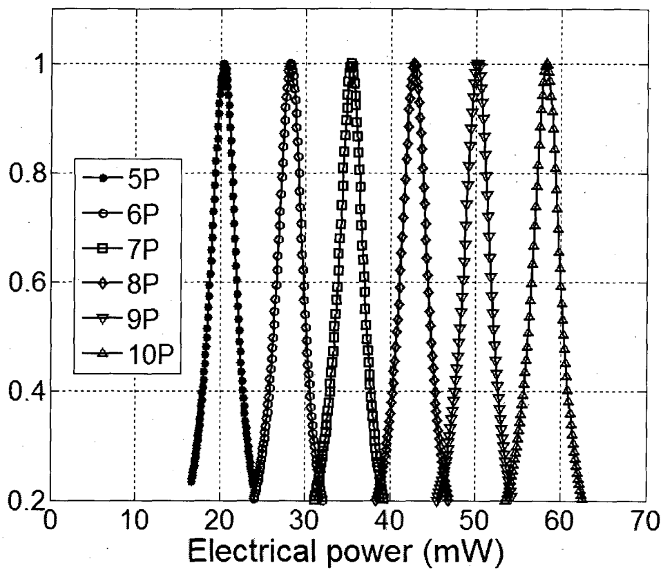
FIG. 5E
