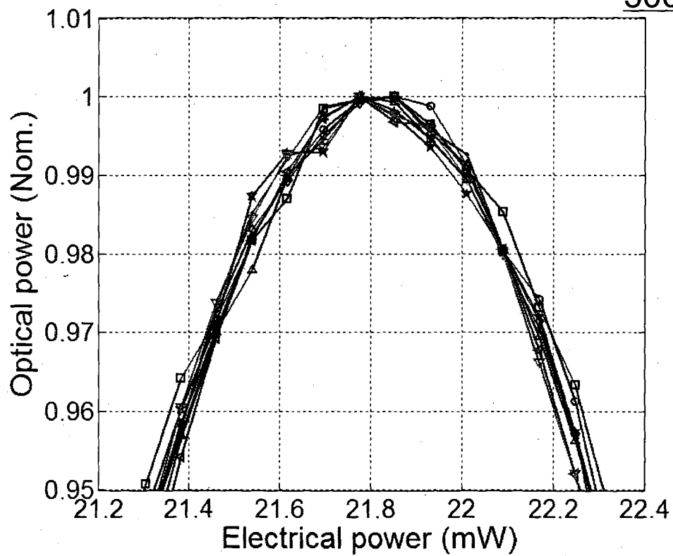
FIG. 5G
