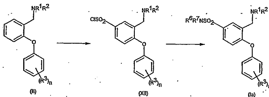
SCHEME 1a
