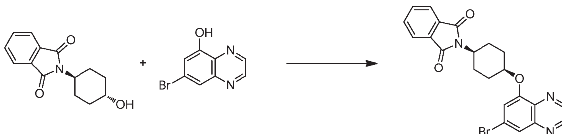
Scheme 10a
