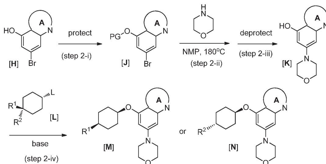
Scheme 2a
