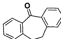
dibenzosuberone
