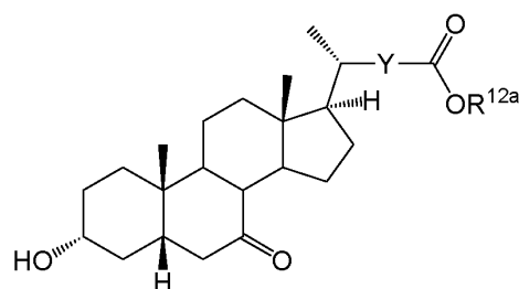
(XVI)
