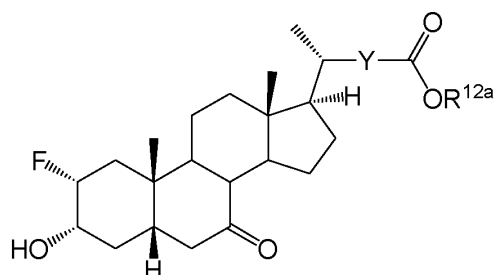
(XIIb)
