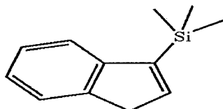
3-(trimethylsilyl)-1H-indene
