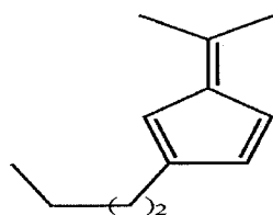
2-(butyl)-6,6-dimethylpentafulvene
