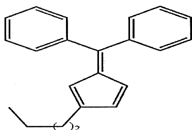
2-(butyl)-6,6-diphenylpentafulvene
