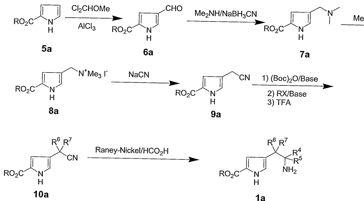
SCHEME 2A
