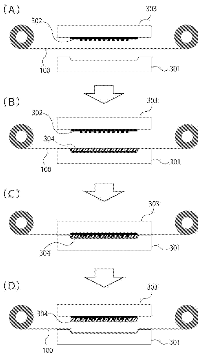
[図4]
