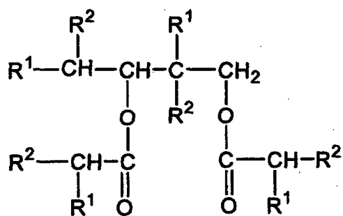
Glycol Diester
