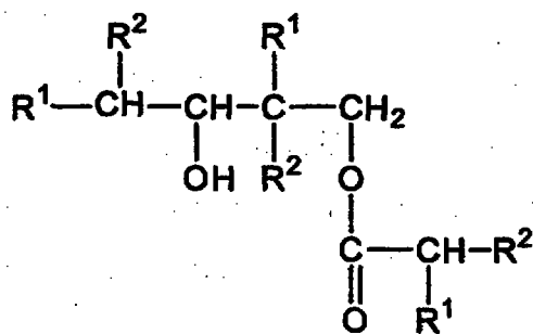
Glycol Monoester
