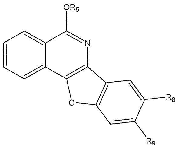
(Ia')
