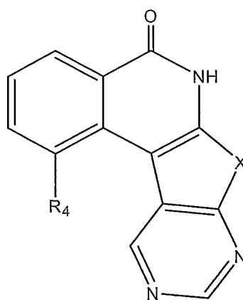
(VIIc')
