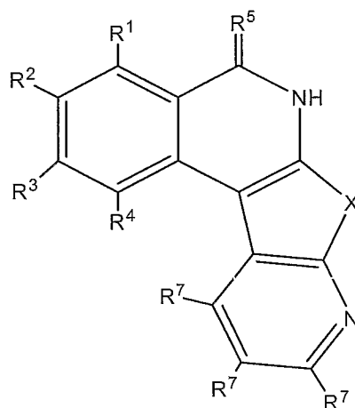
(VIIa)
