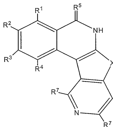
(VIIb)
