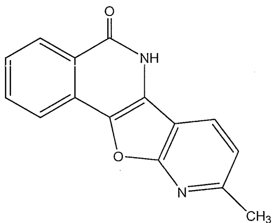
(26a)
