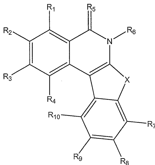
(II)
