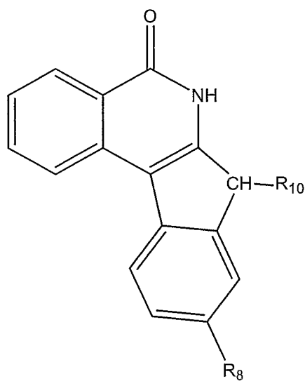
(V')
