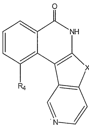
(VIIb')
