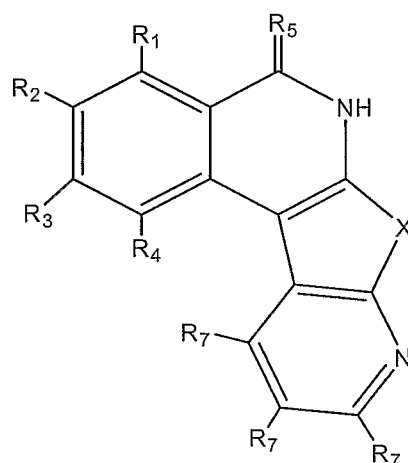
(VIIa)
