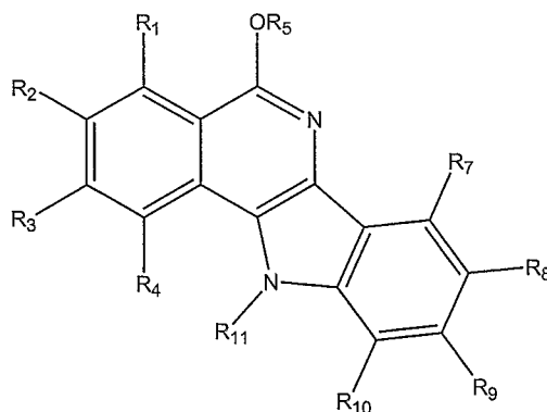
(Ib)
