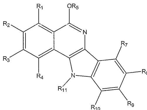
(Ib)
