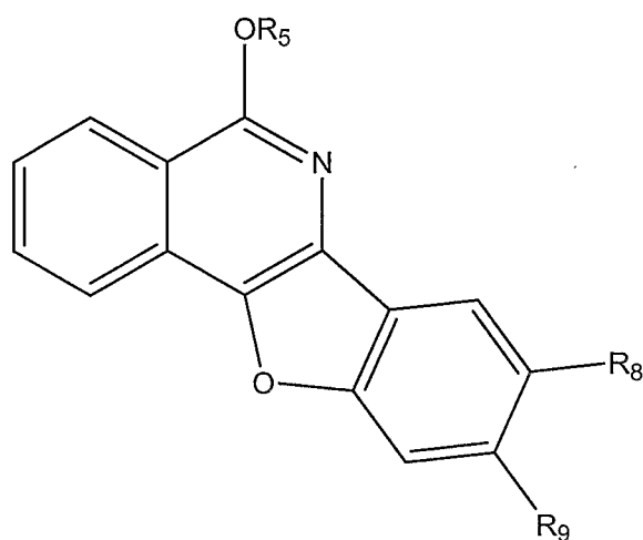
(Ia')
