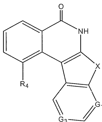
(VII')
