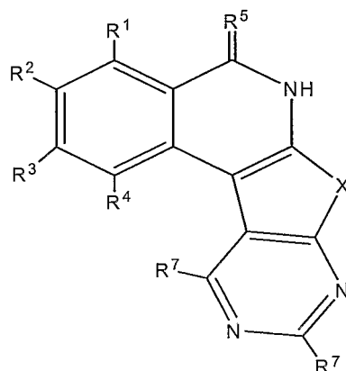
(VIIc)
