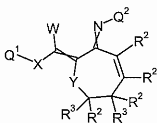
Formula 4.N.4
