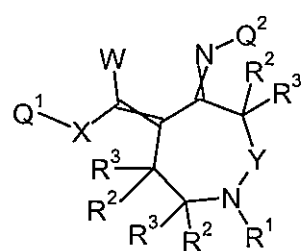
Formula 6.D.9
