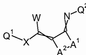
Formula I-a
