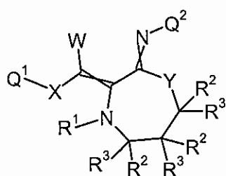
Formula 7.N.1
