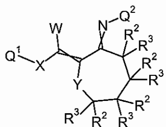
Formula 4.N.1
