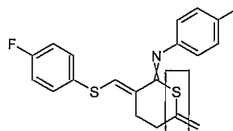
WO2011958963 Example 2-6
