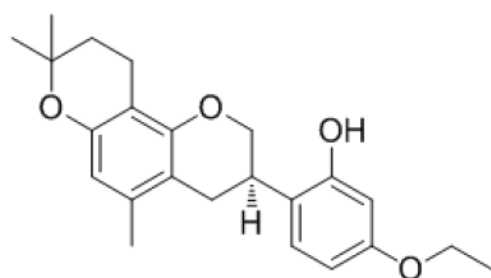
<Compound 9a>
