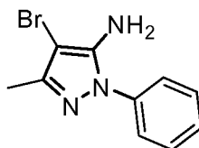
4-bromo-3-methyl-1-phenyl-1H-pyrazol-5-amine
