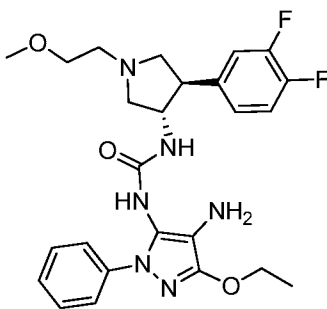
1-(4-amino-3-ethoxy-1-phenyl-1H-pyrazol-5-yl)-3-((3S,4R)-4-(3,4-difluorophenyl)-1-(2-methoxyethyl)pyrrolidin-3-yl)urea
