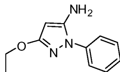
3-ethoxy-1-phenyl-1H-pyrazol-5-amine
