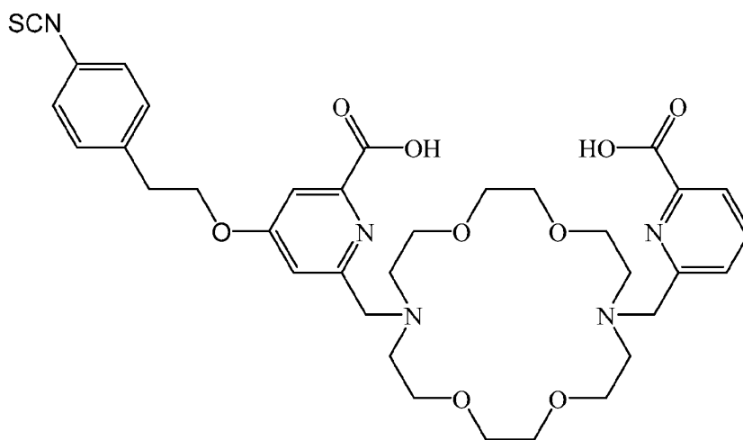
macropa-(OCH 2 CH 2 )-Ph-NCS
