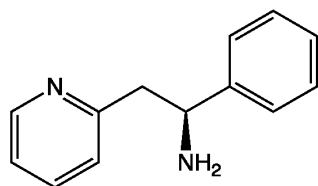
[0006] Lanicemine
