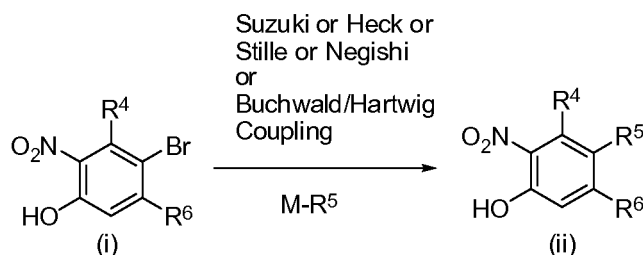
Scheme VI
