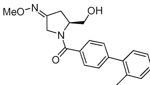
Nolasiban
