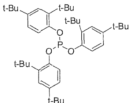
Tris(2,4-di-tert-butylphenyl)phosphite (TDTBPP)
