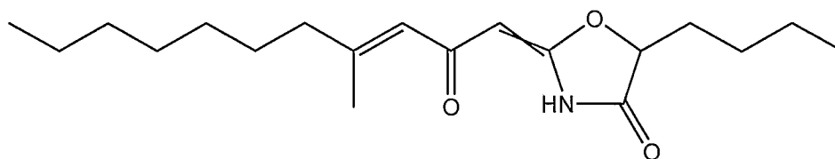
(VI)
