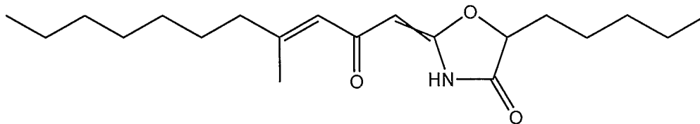
(VII)
