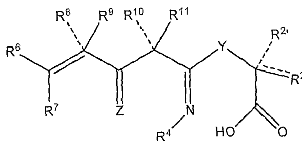
(Va)
