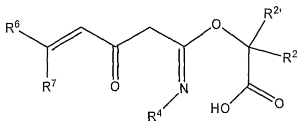
(IVa)
