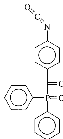
IBPO
