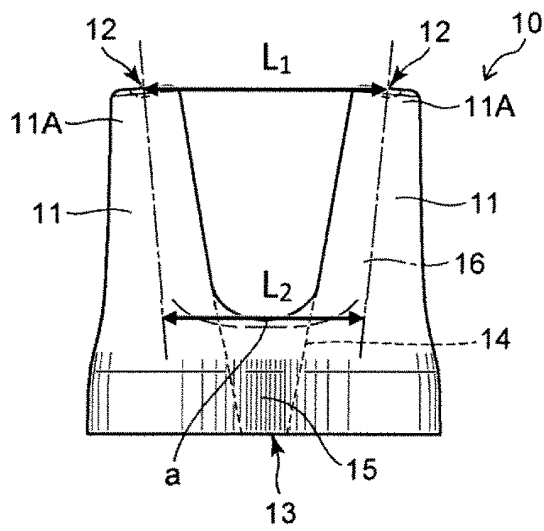
(B) 側方図
