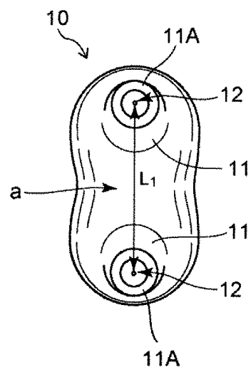
(C) 上方図
