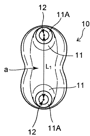
(C) 上方図
