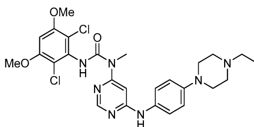
BGJ398;
