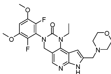
Pemigatinib;
