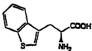
L-(Benzothienyl)-alanine
