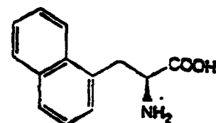
L-1-Nal
