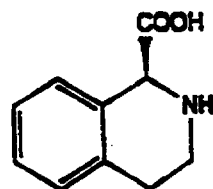
L-Tiq
