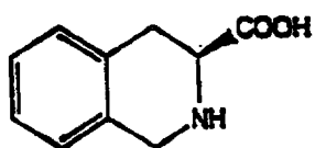
L-Tic
