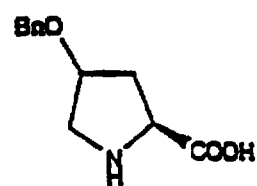
L-4-Hvo (OBn)
