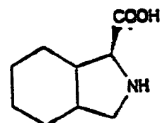
L-Oic
