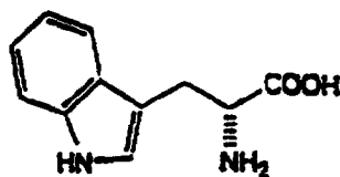
D-Trp
