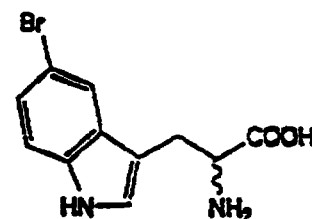
DL-5-Br-Trp
