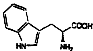
L-Trp
