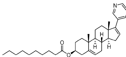
abiraterone decanoate.
