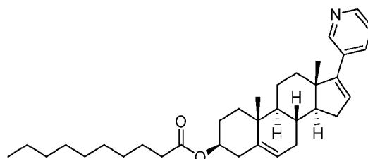
abiraterone decanoate.
