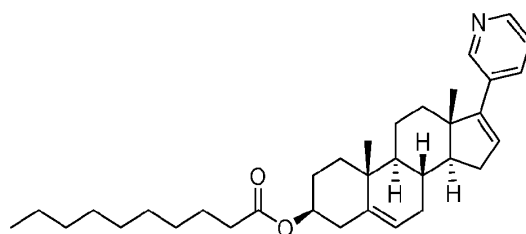
abiraterone decanoate.
