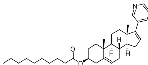
abiraterone decanoate.
