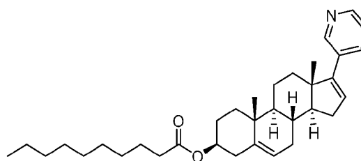
abiraterone decanoate.
