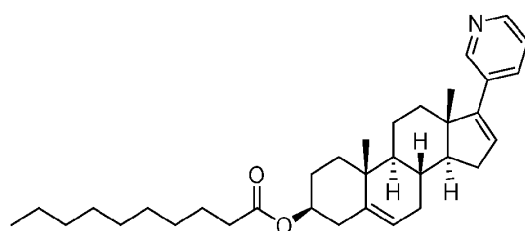
abiraterone decanoate.
