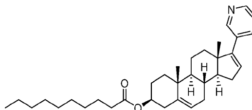
abiraterone decanoate.
