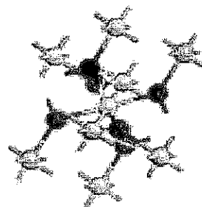
Rutile
