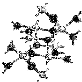
Brookite
