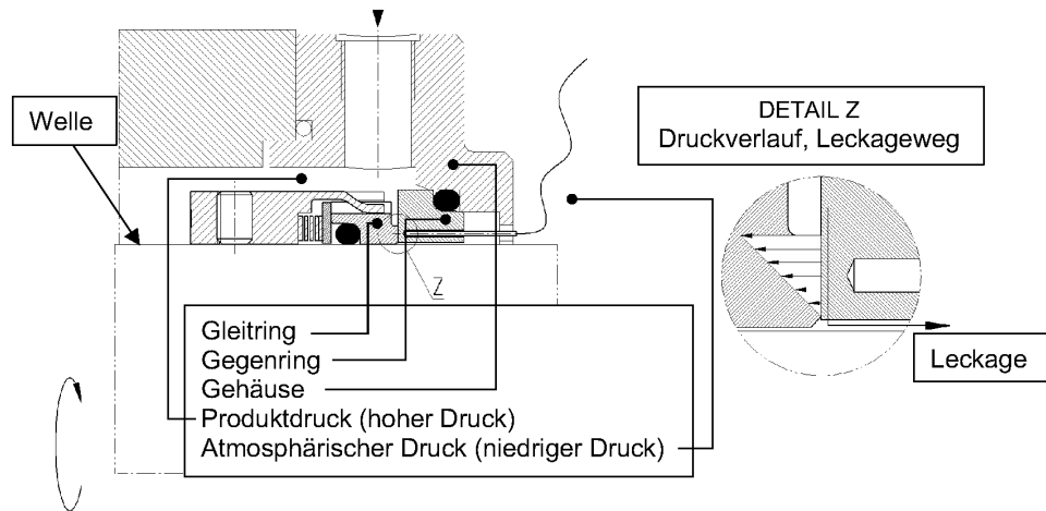
Figur 2 Anordnung Gleitringdichtung mit Temperaturmessung
