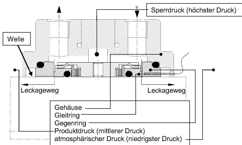
Figur 3 Anordnung gesperrte Doppeldichtung
