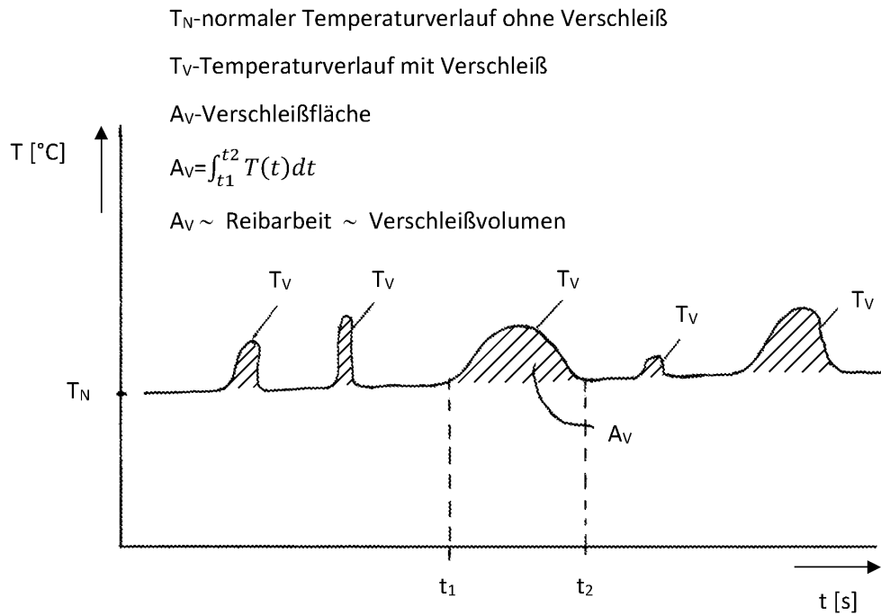
Figur 4 Temperaturverlauf
