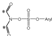
N-(carbonylcarbamido) aryl sulfate moiety
