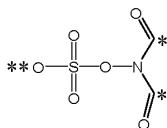
N-(carbonylcarbamido) sulfate moiety
