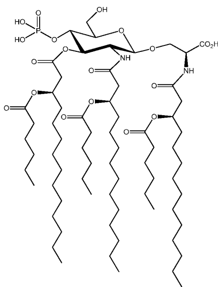
CRX-526
