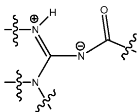
Formula (D)
