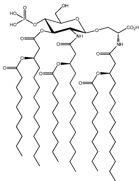
CRX 547
