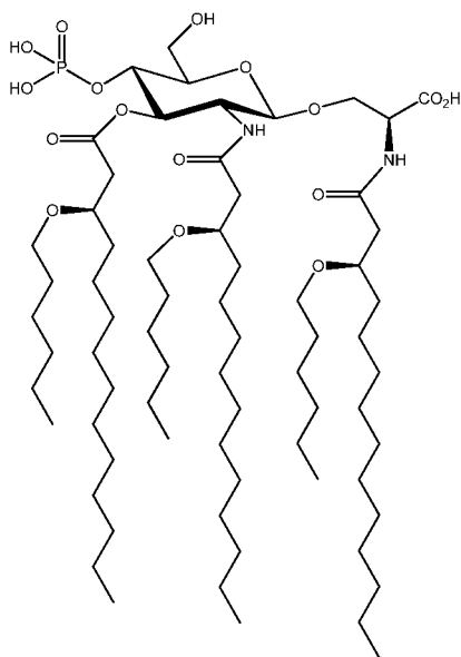
CRX 602
